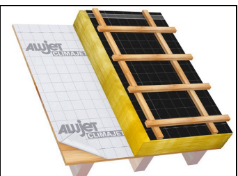
Abb. 5: unter Aufdachdämmung
